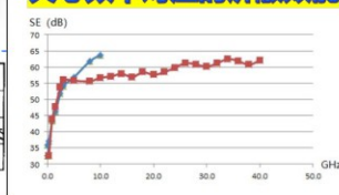
关心频率对应的屏蔽效能
