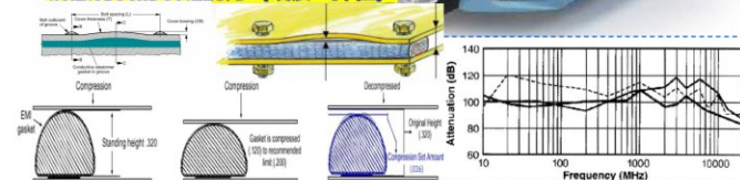
屏蔽材料的压缩能力 (硬度&弹性)
